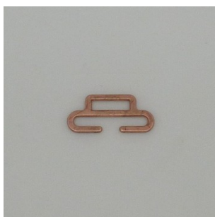
08804-00-07 Größe: ca. 24x11 mm Innenmaß: 20 mm Abbildung: verkupfert
