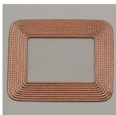
05009-00-00 Größe: ca. 60x47 mm Abbildung: verkupfert
